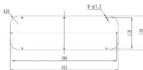
2号凸台封板
