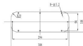
3号凸台封板
