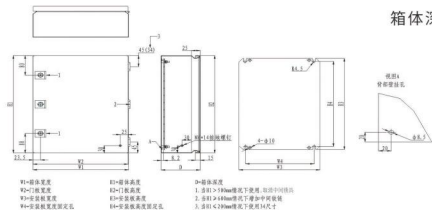
箱体深度
