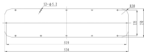
1号凸台封板
