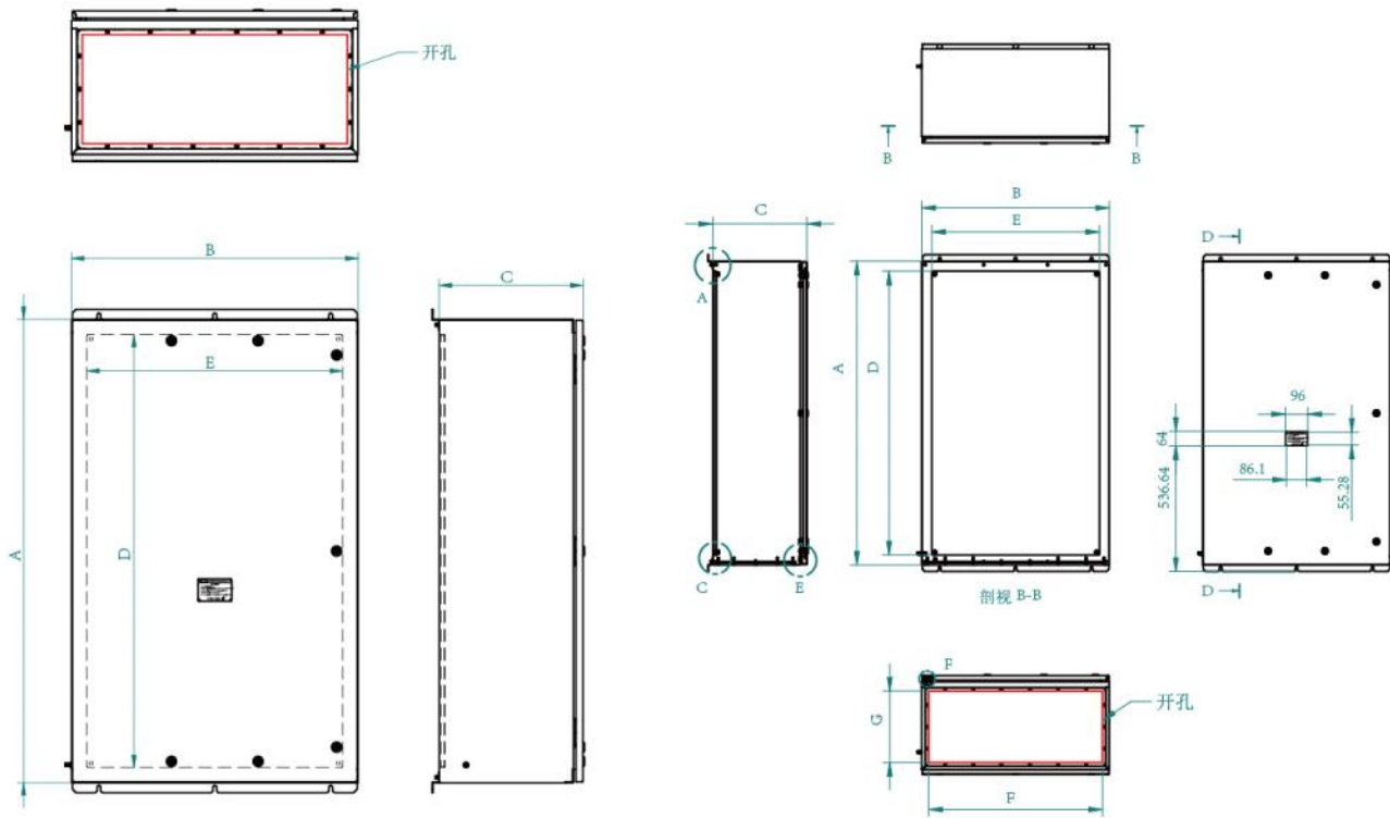
细节图 Details
