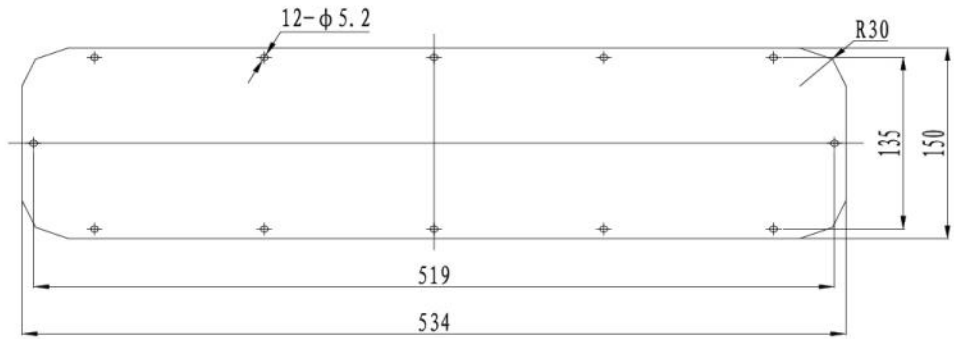
1号凸台封板
