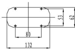
5号凸台封板
