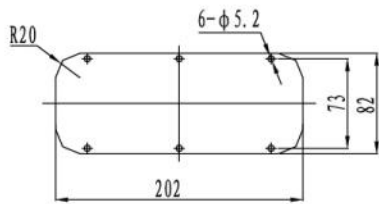
4号凸台封板
